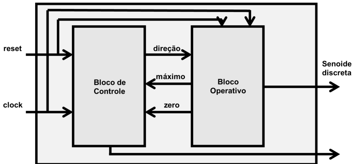
Figura 16 – Diagrama de blocos da conexão dos blocos operativo e controle
