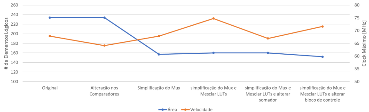
Figura 19 – Resultados da implementação em FPGA
