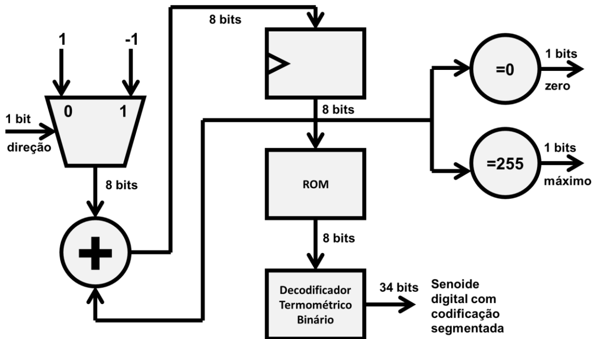
Figura 14 – Diagrama de blocos do bloco operativo
