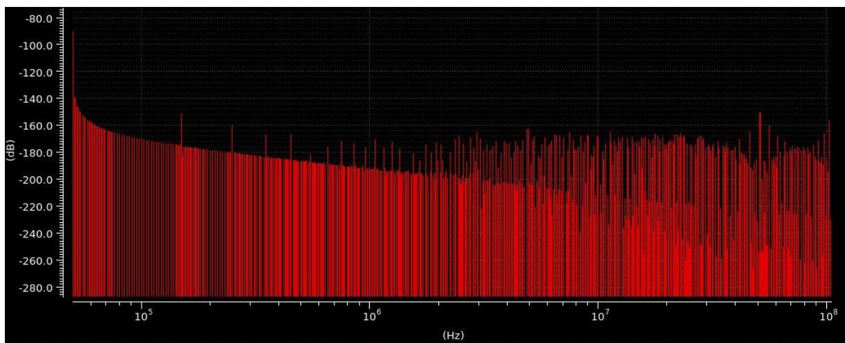
Figura 22 – Espectro obtido por FFT do resultado da simulação de sinais mistos
