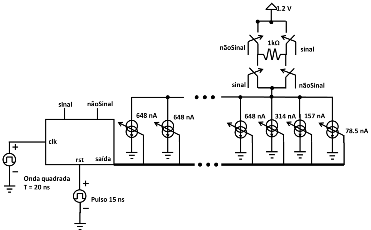
Figura 20 – Testbench para o sistema
