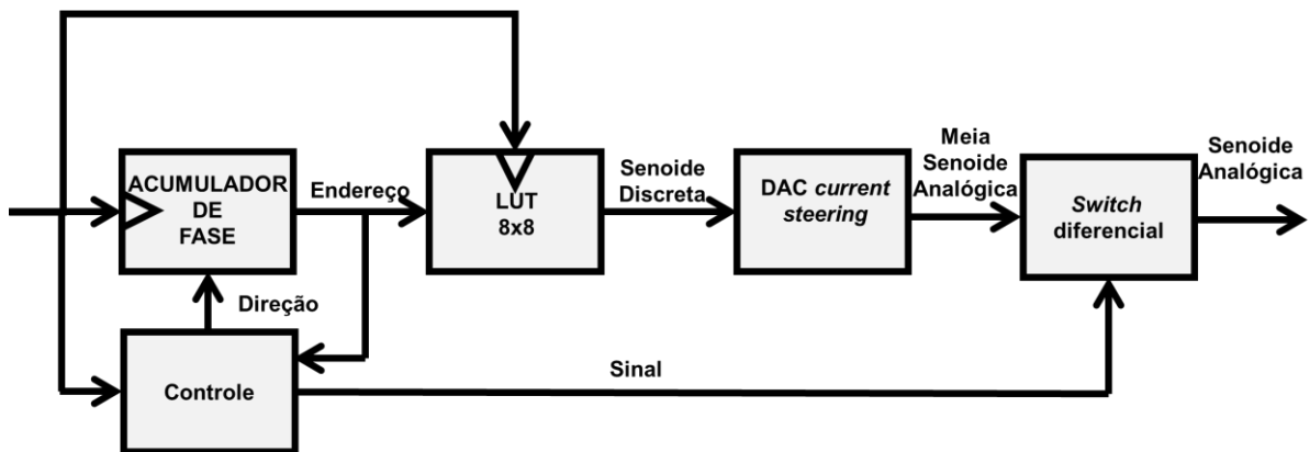
Figura 13 – Diagrama de blocos do DDS específico da aplicação
