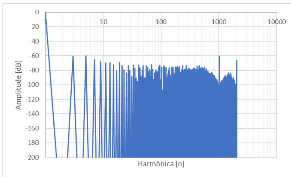
Figura 11 – Espectro para a representação de 8 bits
