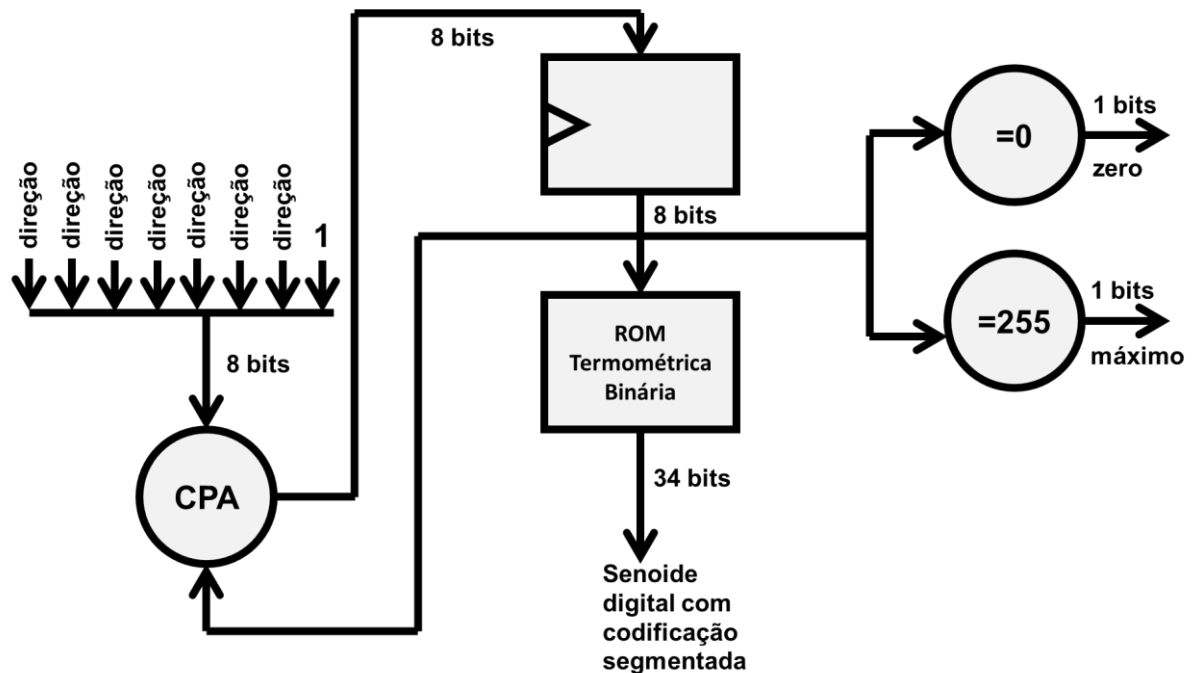
Figura 17 – Bloco Operativo otimizado
