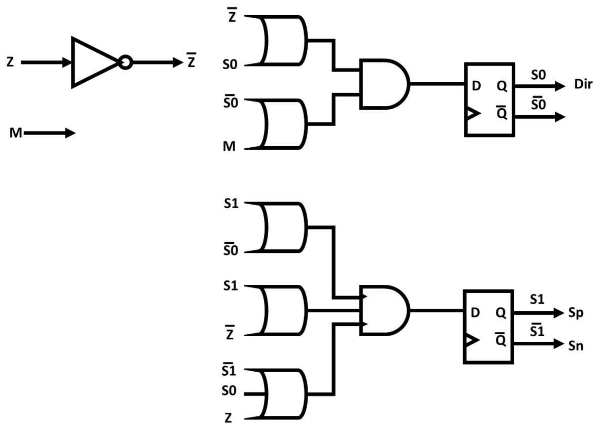
Figura 18 - Ilustração da lógica otimizada do controle
