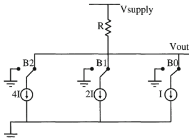
Figura 5 – Exemplo de arquitetura de DAC current steering
