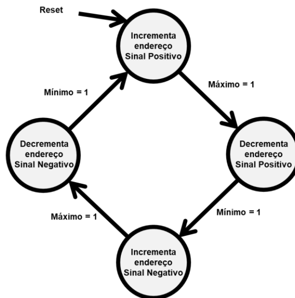
Figura 15 – FSM do bloco de controle
