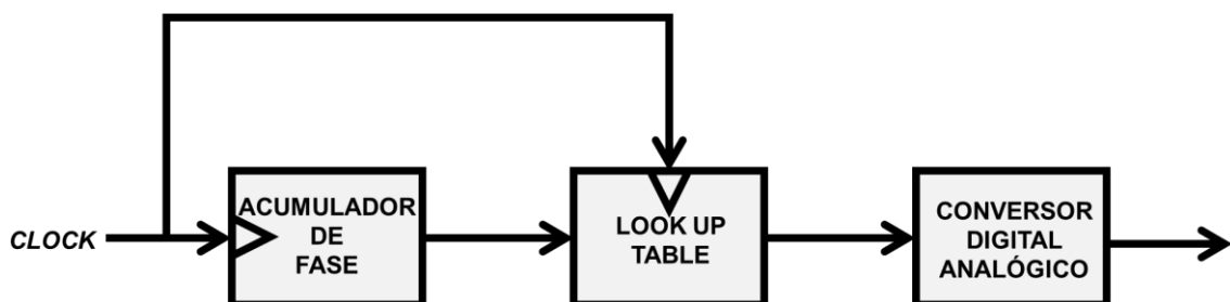
Figura 4 – Diagrama de blocos de um DDS
