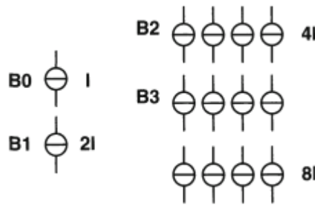
Figura 7 – Exemplo da implementação das fontes de corrente em arquitetura segmentada
