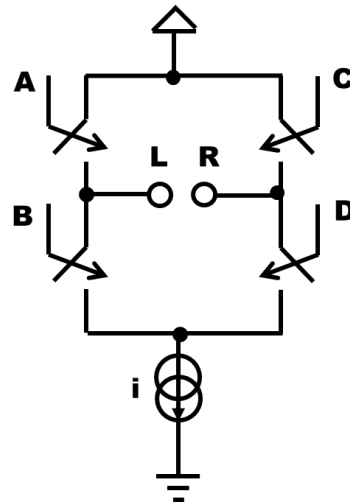
Figura 6 – Esquemático básico de um circuito de ponte-H
