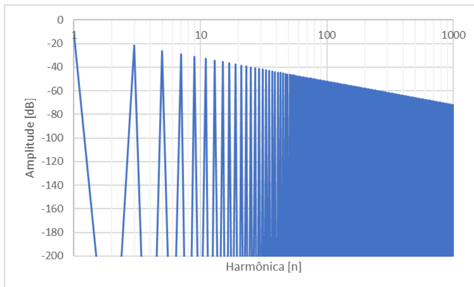
Figura 9 – Espectro da forma de onda utilizando apenas um bit
