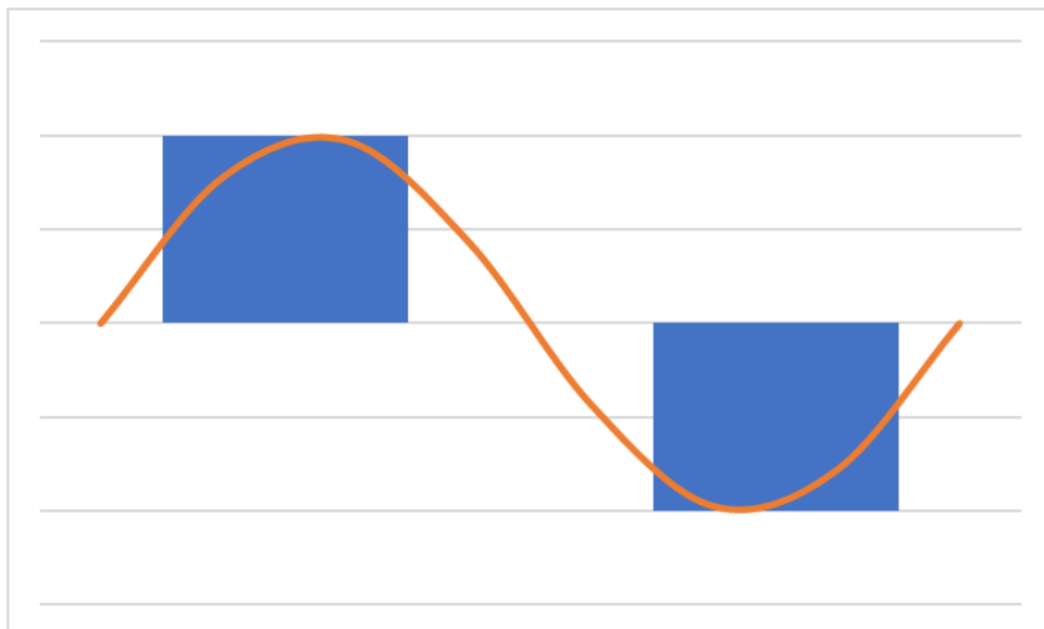
Figura 8 – Exemplo de discretização da senoide utilizando apenas um bit
