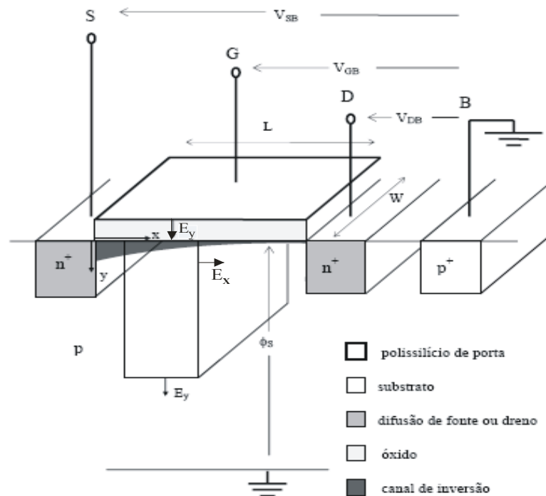
Figura 3-1: Estrutura física de um transistor MOS.
