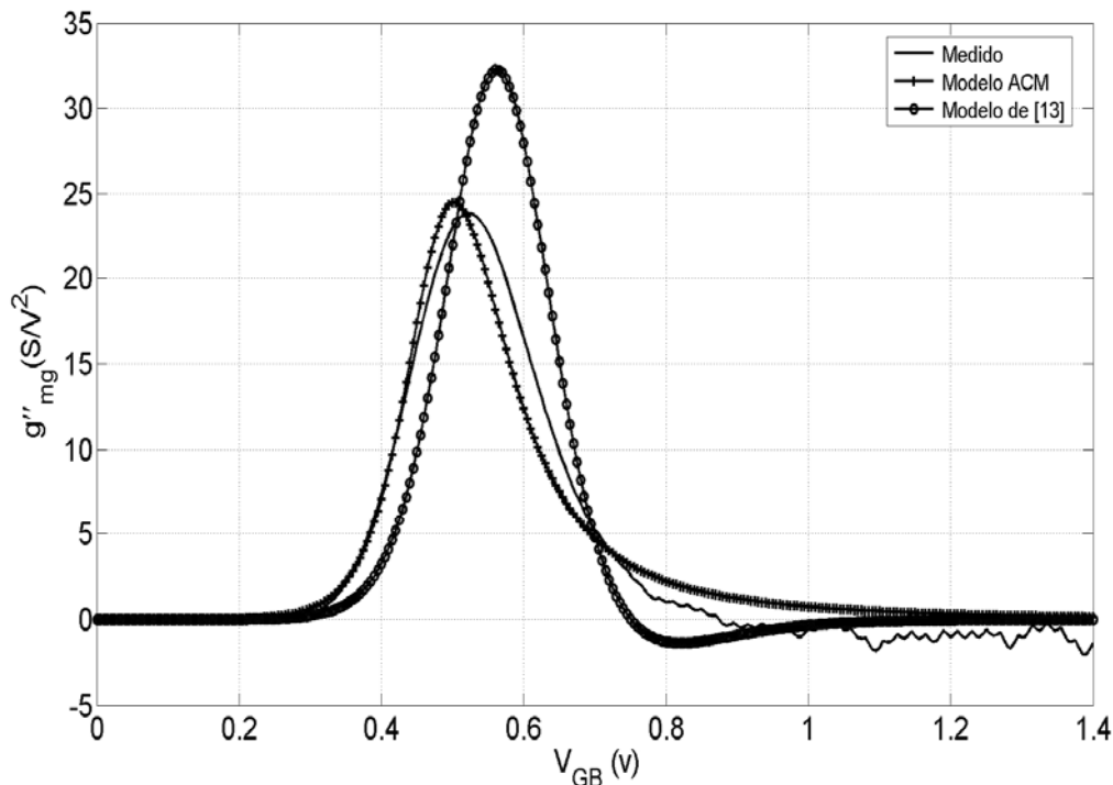
Figura 4-5: Comparação entre modelos e medida.
