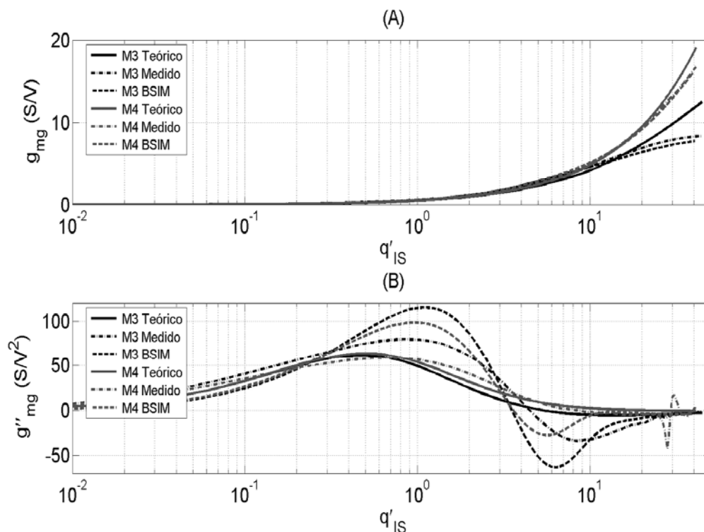
Figura 5-3: (A) g_{mg} e (B) g_{mg}'' para os transistores da tecnologia TSMC 0.35 \mu m .
