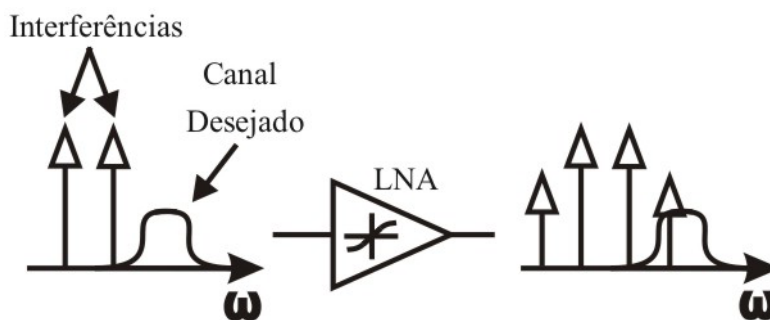
Figura 2-3: Problema da intermodulação em forma esquemática.
